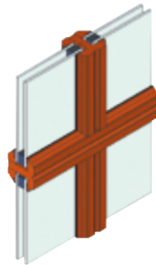
Petits bois mortaisés Petit bois mortaisé largeur 53 mm. Il est assemblé par tenon dans le vantail. C'est le petit bois traditionnel adapté aux normes actuelles.
